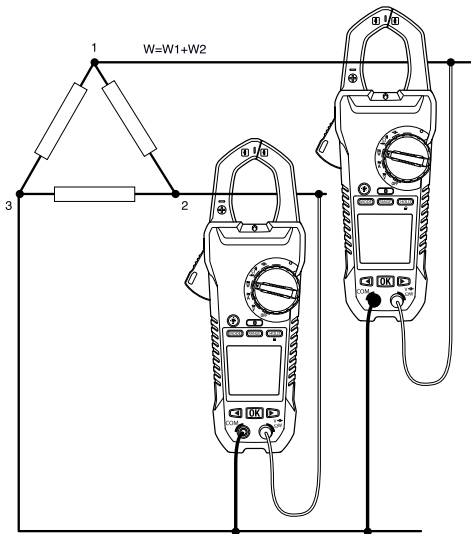
Figuur 5.3 Meting aan driefasige driedraadse schakelingen
