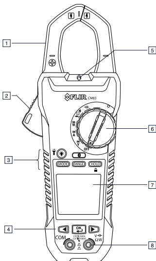
Figuur 4.1 Vooraanzicht
