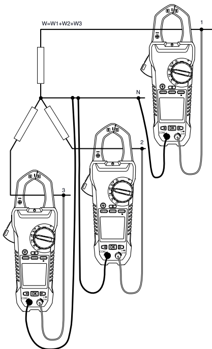
Figuur 5.4 Meting aan driefasige vierdraadse schakelingen
