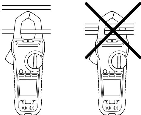
Figuur 5.1 Juiste en verkeerde meetopstelling
